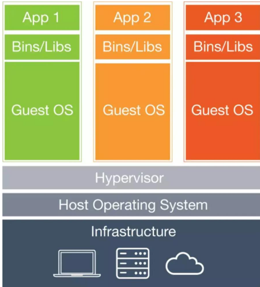
虚拟化架构
