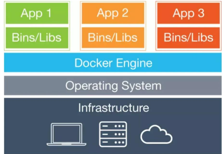
容器架构
