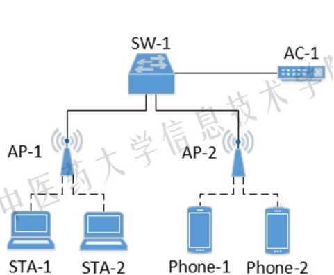
图 7-1 网络拓扑 1
