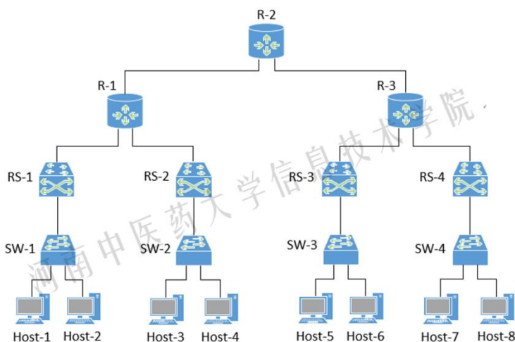
图 3-1 网络拓扑
