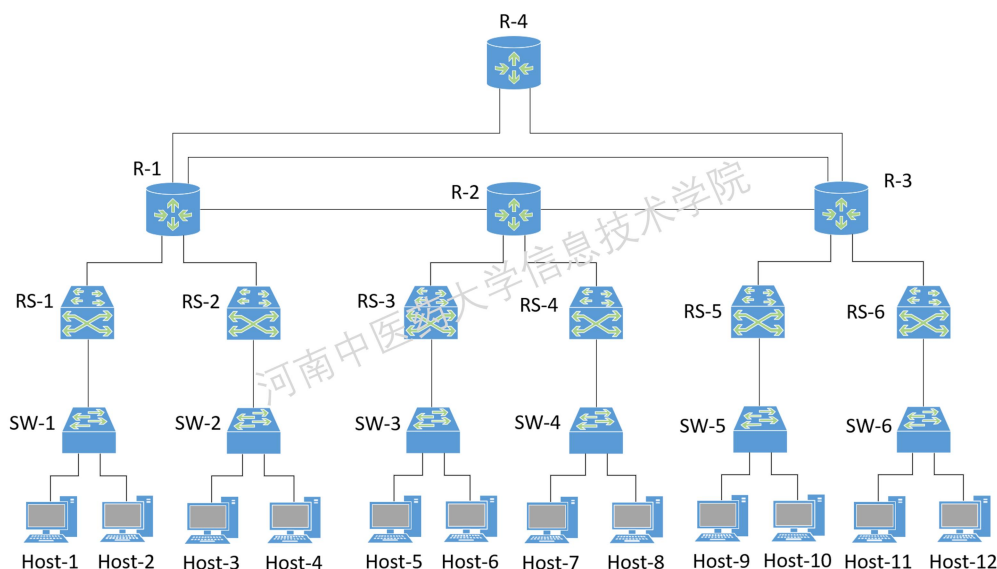
图 4-1 网络拓扑
