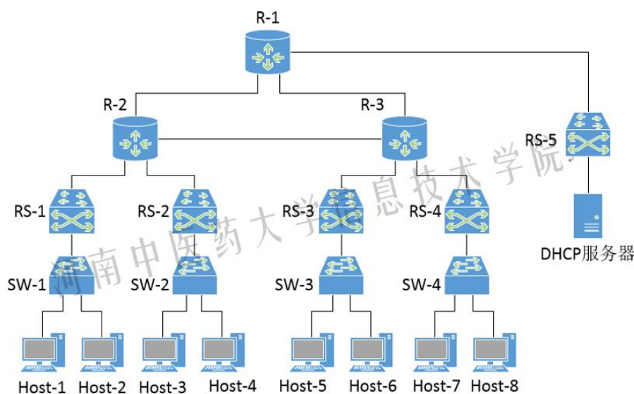
图 6-1 网络拓扑
