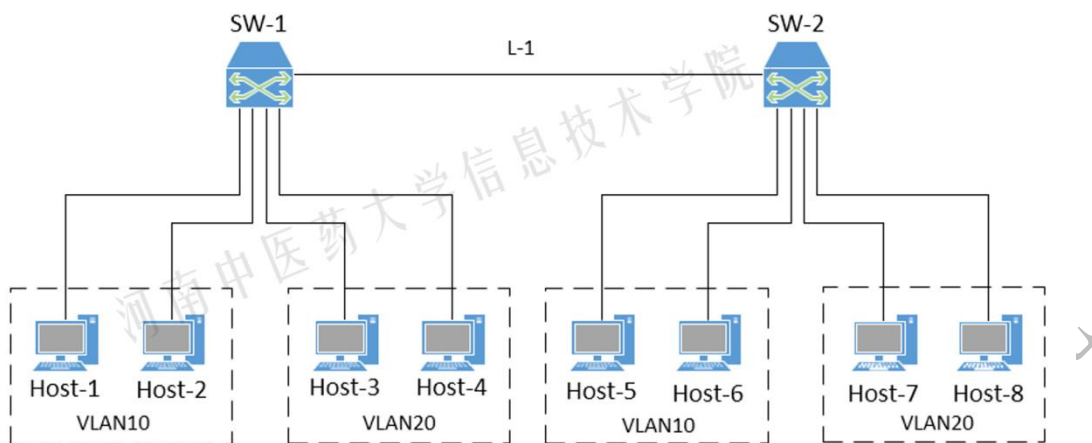
图 1 任务 1 拓扑
