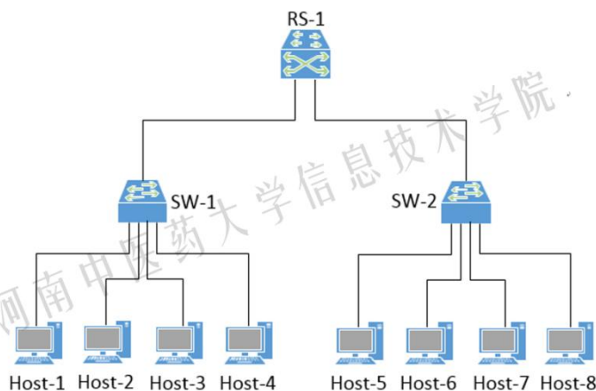
图 2 任务 2 拓扑
