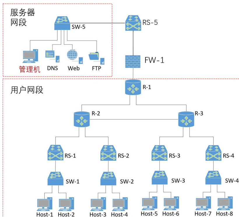
图 8-1 网络拓扑
