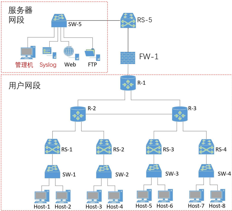
图 9-1 网络拓扑
