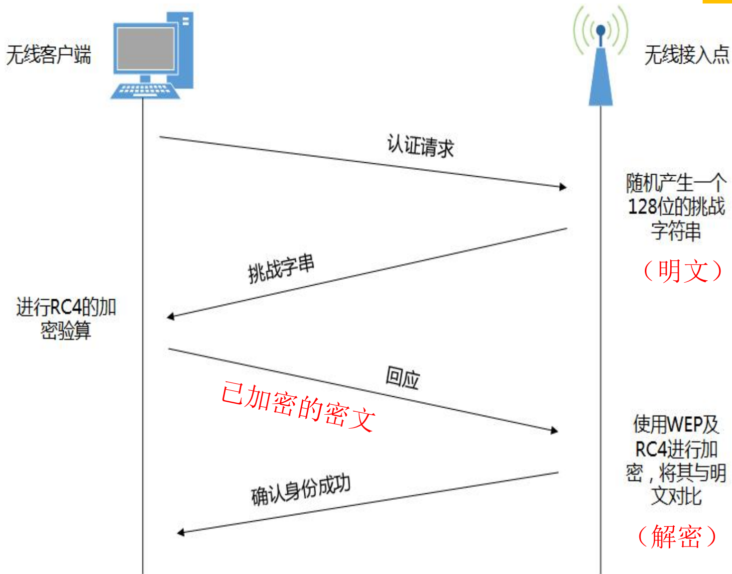
WEP加密的验证及加密过程
