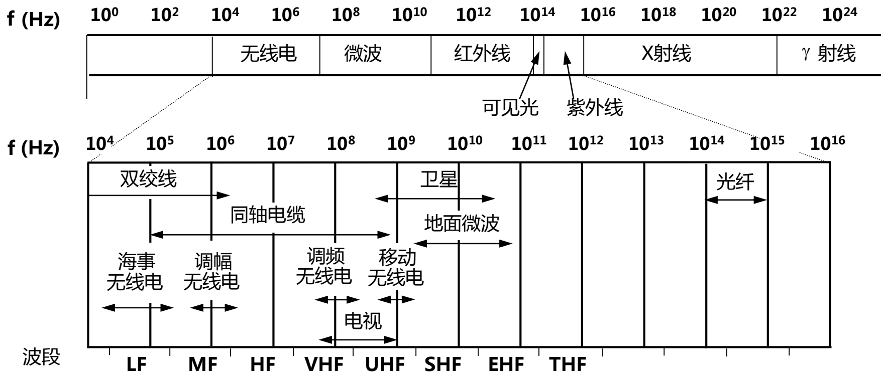
电信领域使用的电磁波的频谱
