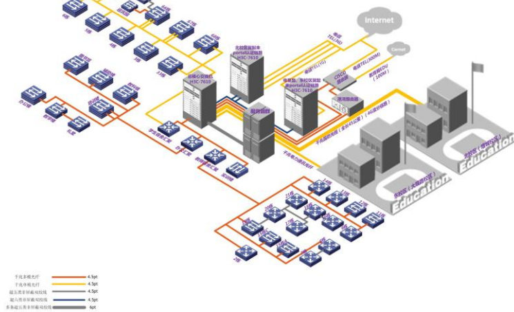
广东农工商职业技术学院 粤垦路校区网络拓扑图
