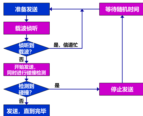
CSMA/CD 协议工作流程
