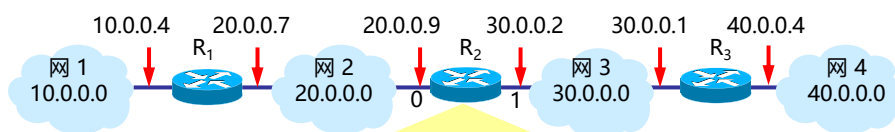
路由器R 2 的路由表
