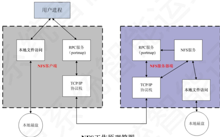
NFS工作原理简图
