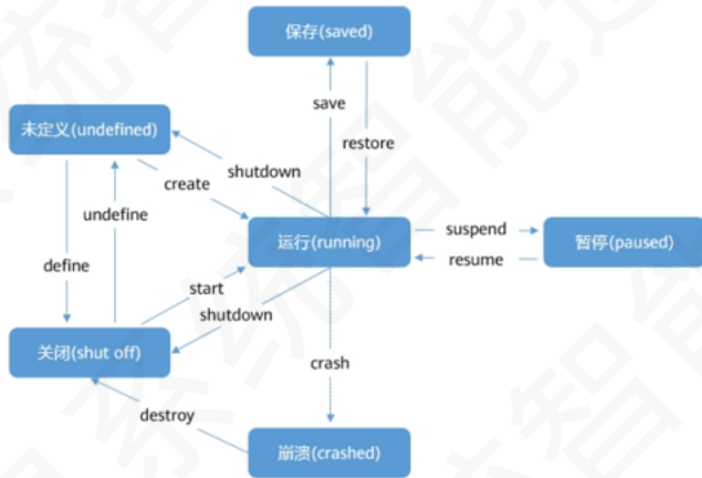
KVM虚拟机状态转化图
