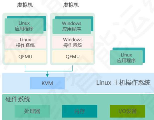
KVM架构图
