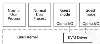
KVM结构
