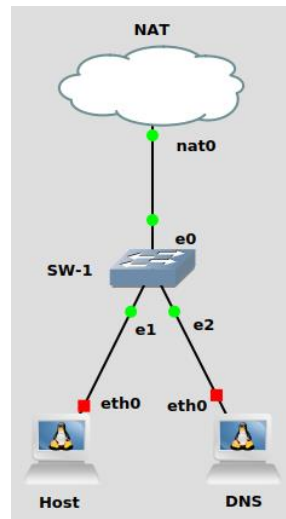
图 6-7 实现网络
