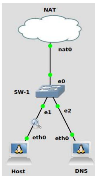
图 6-10 抓包位置设置
