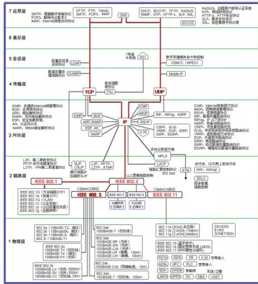
常用网络通信协议结构图
