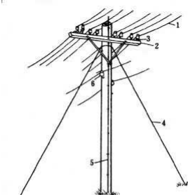
明线线路图 1 导线 2 横担 3 直螺帽 4 拉线 5 电杆 6 绝缘子
