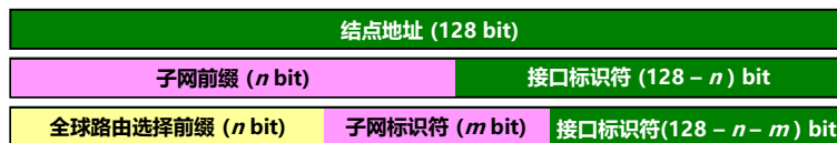
IPv6 单播地址的几种划分方法
