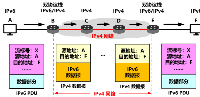
使用隧道技术进行从 IPv4 到 IPv6 的过渡
