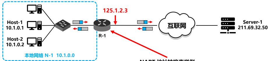
NAPT 地址转换表举例
