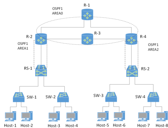
图 5-5 网络拓扑
