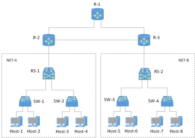
图 5-1 网络拓扑
