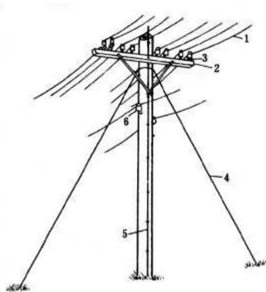
明线线路图
