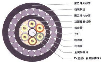
光缆剖面的示意图
