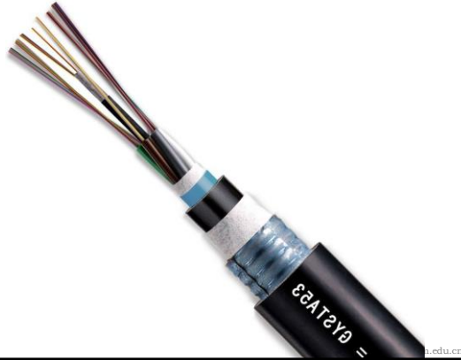
光缆剖面的示意图
