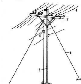
明线线路图 1 导线 2 横担 3 直螺帽 4 拉线 5 电杆 6 旁接避雷电子
