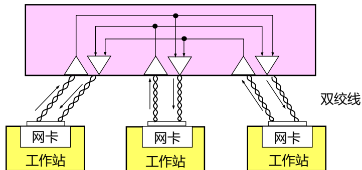
具有三个接口的集线器的逻辑结构
