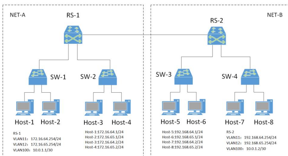
图 1-22 园区网拓扑
