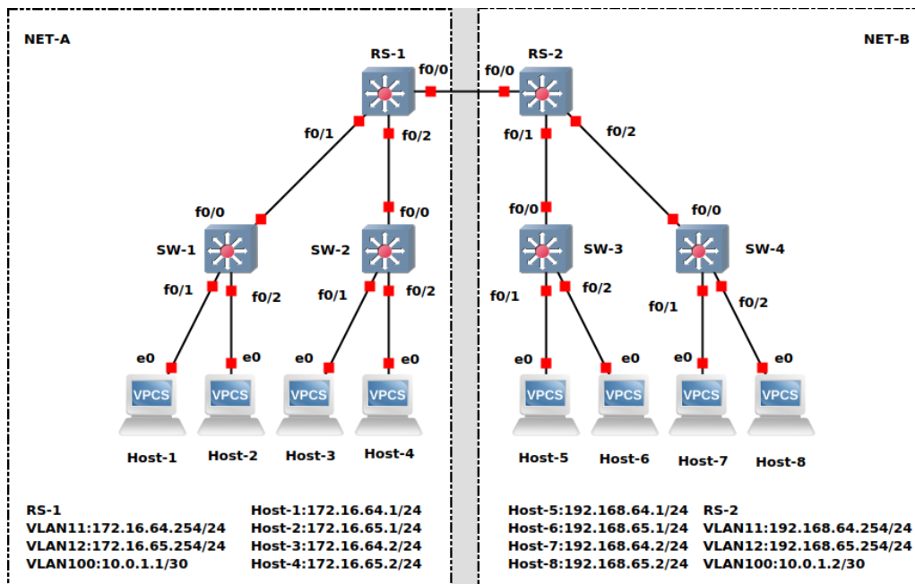
图 1-23 园区网拓扑
