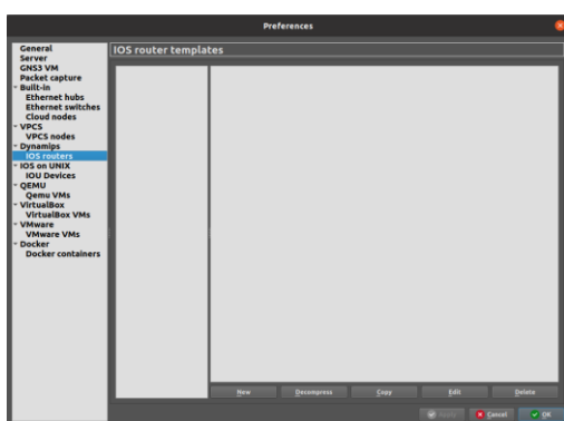
图 1-3 添加镜像
