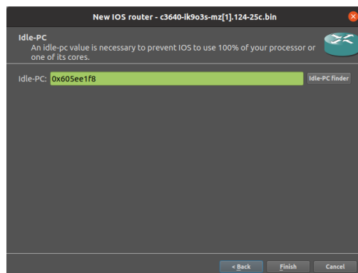
图 1-8 配置 Idle-PC
