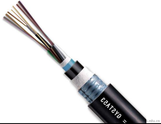
光缆剖面的示意图
