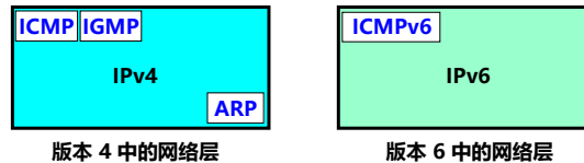
新旧版本中的网络层的比较
