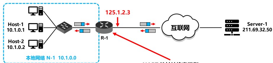
NAPT 地址转换表举例
