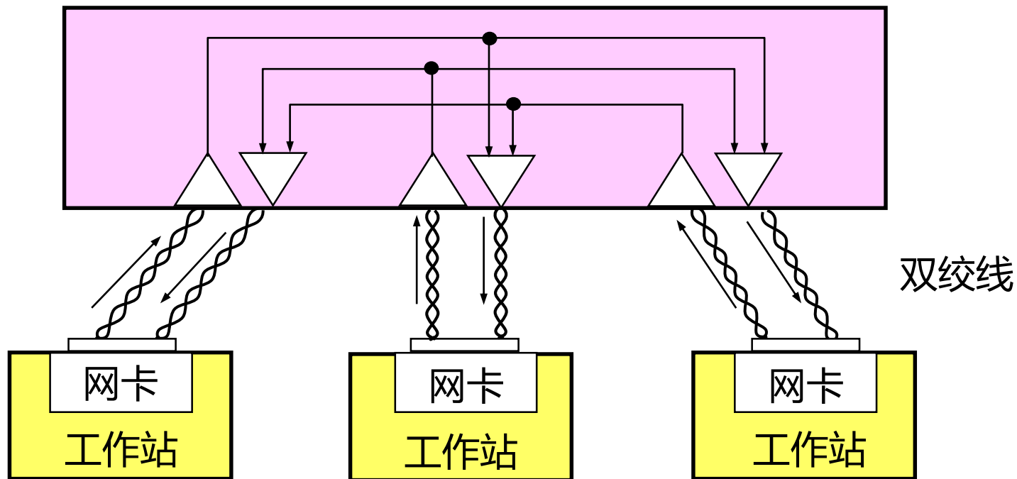
具有三个接口的集线器的逻辑结构
