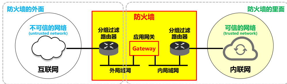
防火墙在互连网络中的位置
