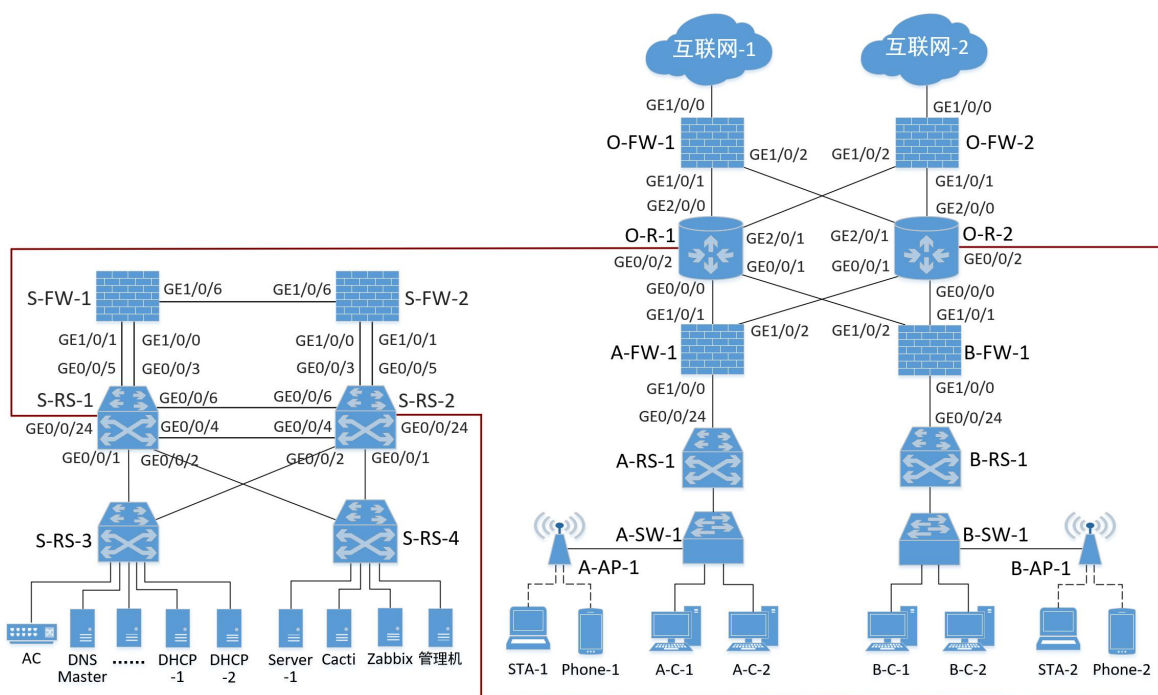
图 2 加入防火墙后的拓扑设计
