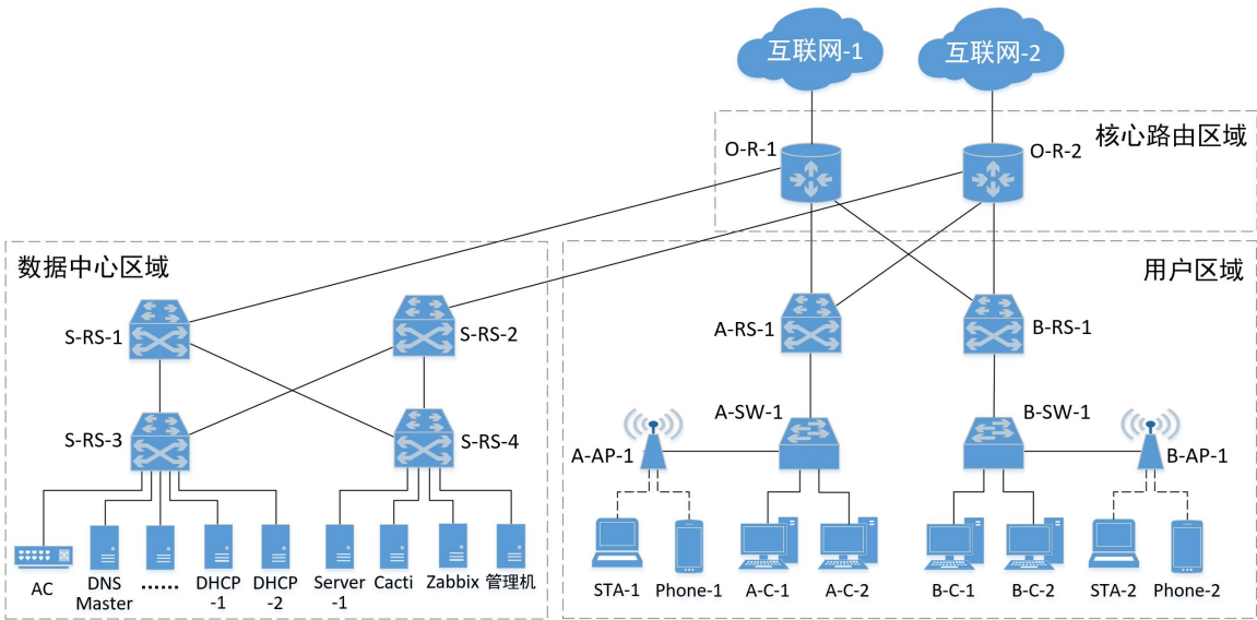
图 1 未加入安全设计的网络拓扑
