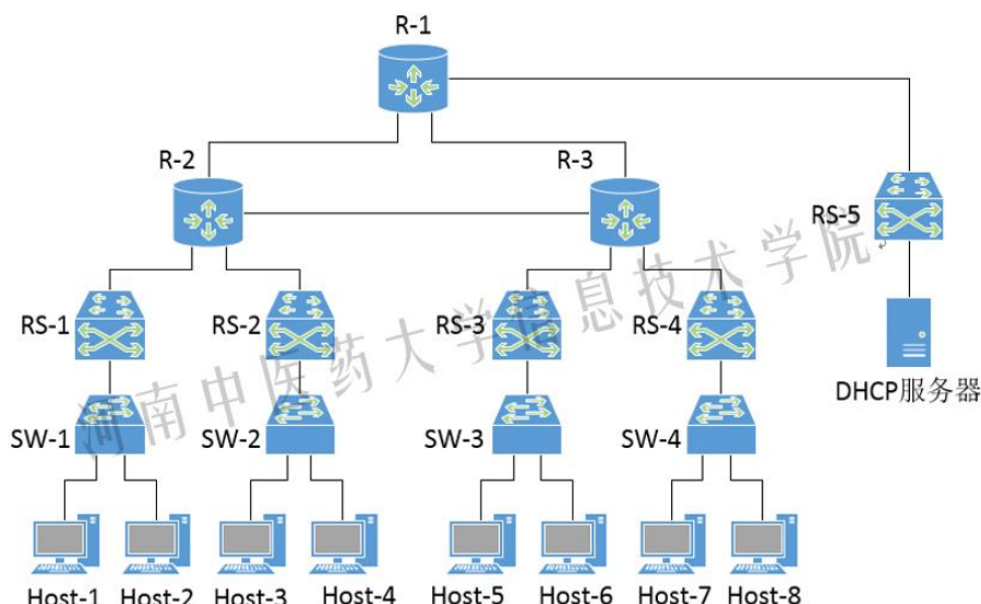
图 6-1 网络拓扑
