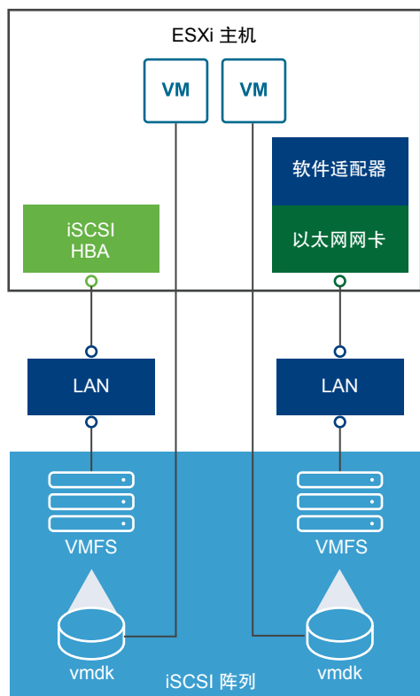
图 2-3. iSCSI 存储
