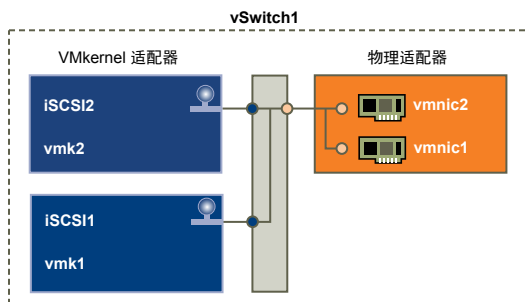
图 11-2. 单个 vSphere 标准交换机上的一对一适配器映射
