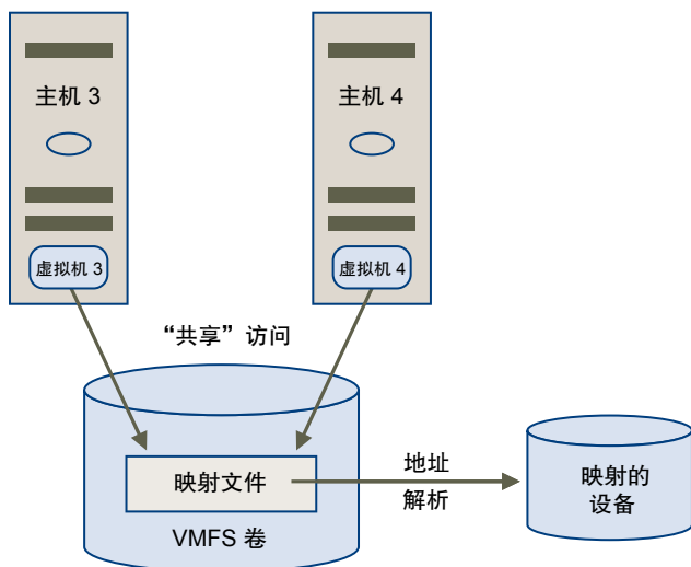
图 19-3. 从群集虚拟机进行访问
