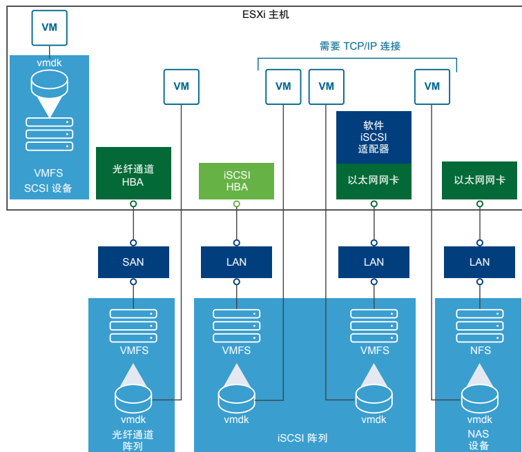
图 2-6. 访问不同类型存储的虚拟机
