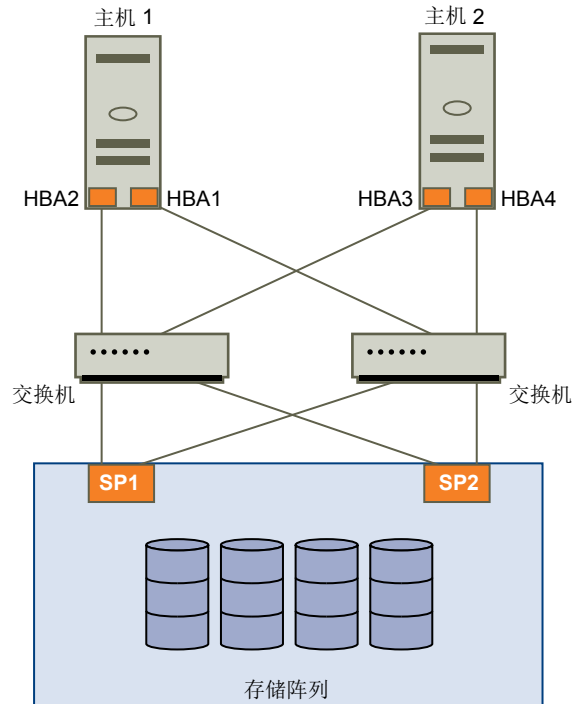
图 18-1. 多路径和光纤通道故障切换
