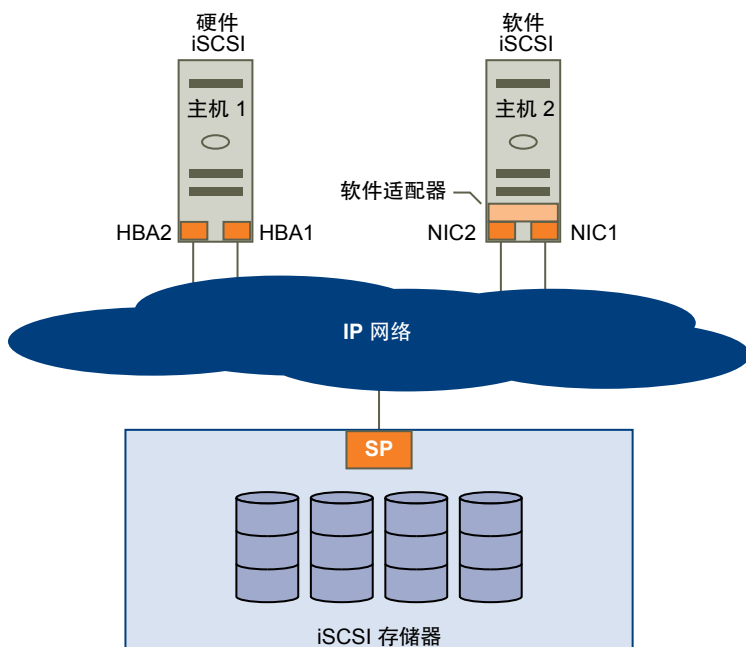
图 18-2. 基于主机的路径故障切换
