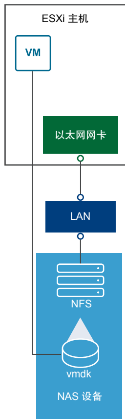
图 2-4. NFS 存储
