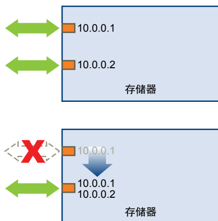
图 18-4. 端口重新分配
