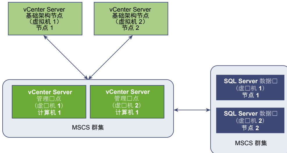
图 5-1. 实现 vCenter Server 高可用性的 MSCS 群集
