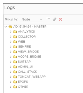
图 4-1. 日志
