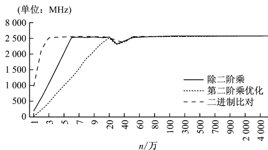
图 9 消耗 CPU 频率使用量对比图
