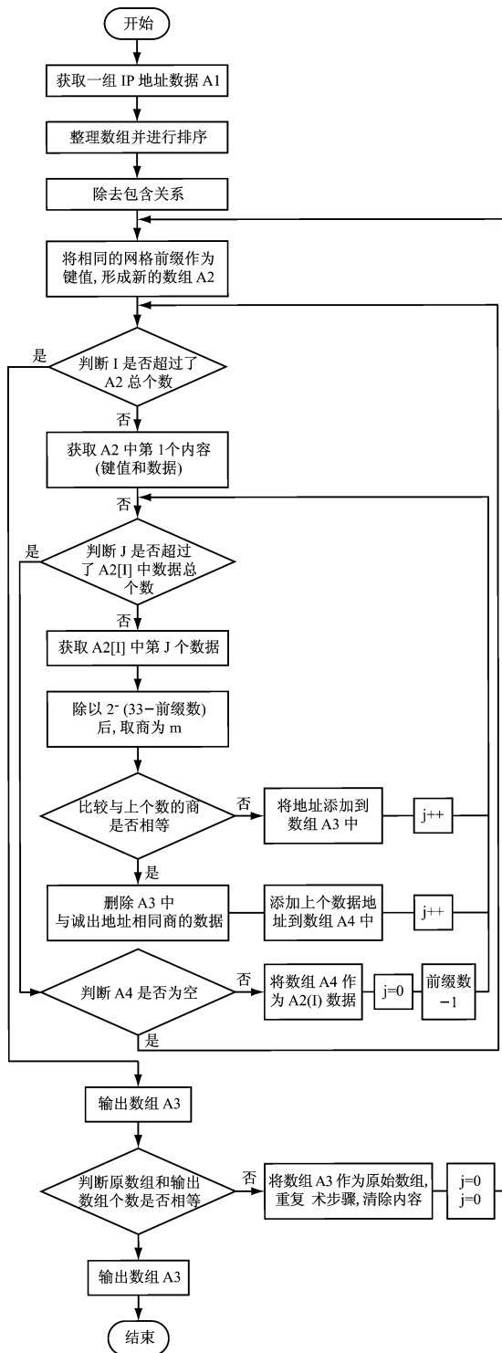
图 2 排序流程
