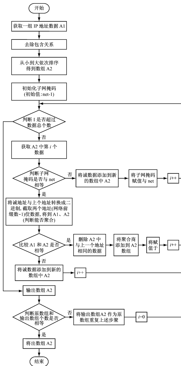
图 4 “二进制比对”聚合算法过程
